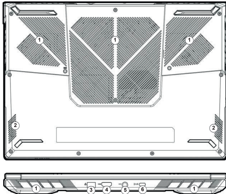
Figura 7 Vistas inferior e traseira
