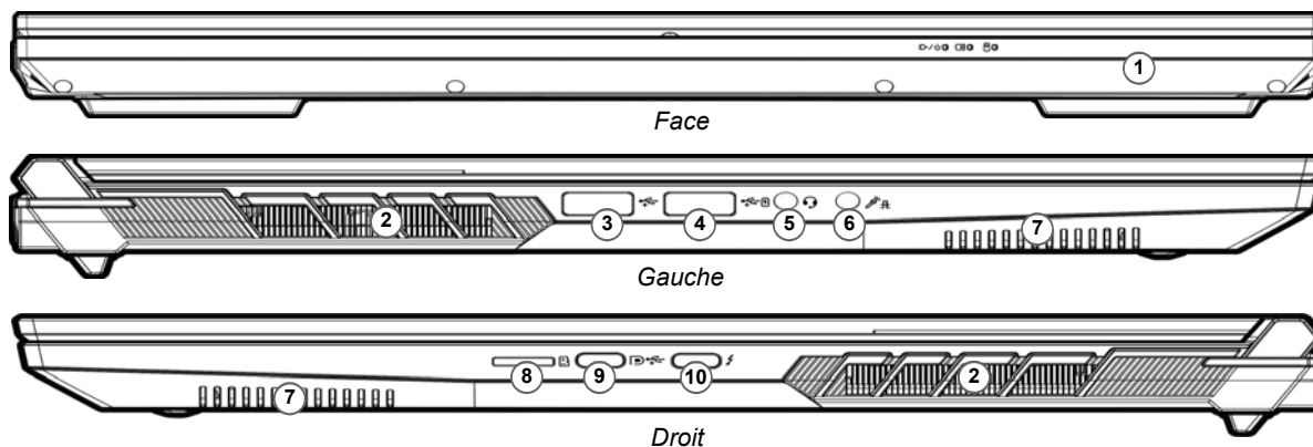
Figure 4 - Vues de face, gauche et droite (Modèle B)
