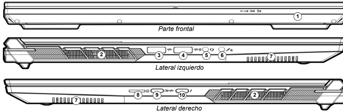
Figura 4 - Vistas frontal, izquierda y derecha (Modelo B)
