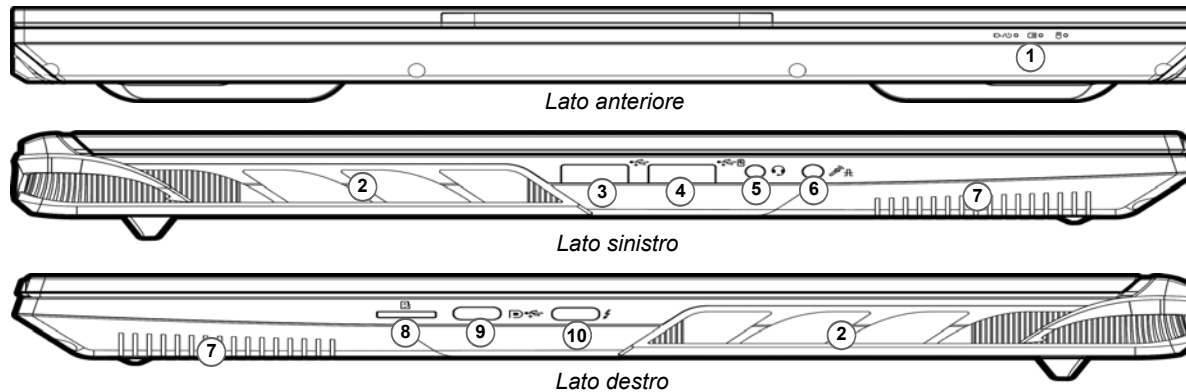
Figura 3 - Vista anteriore, sinistra e destra (Modello A)
