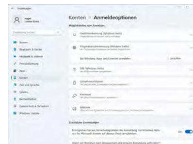
Abb. 13 - Konten - Anmeldeoptionen
