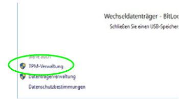
Abb. 15 BitLocker-Laufwerkverschlüsselung (TPM-Verwaltung)
